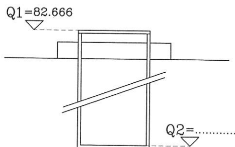
Sezione scala 1:50
